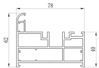
Frame ZDM7801
