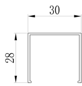
Channel ZDM7807
