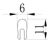
Rail ZDM7802
